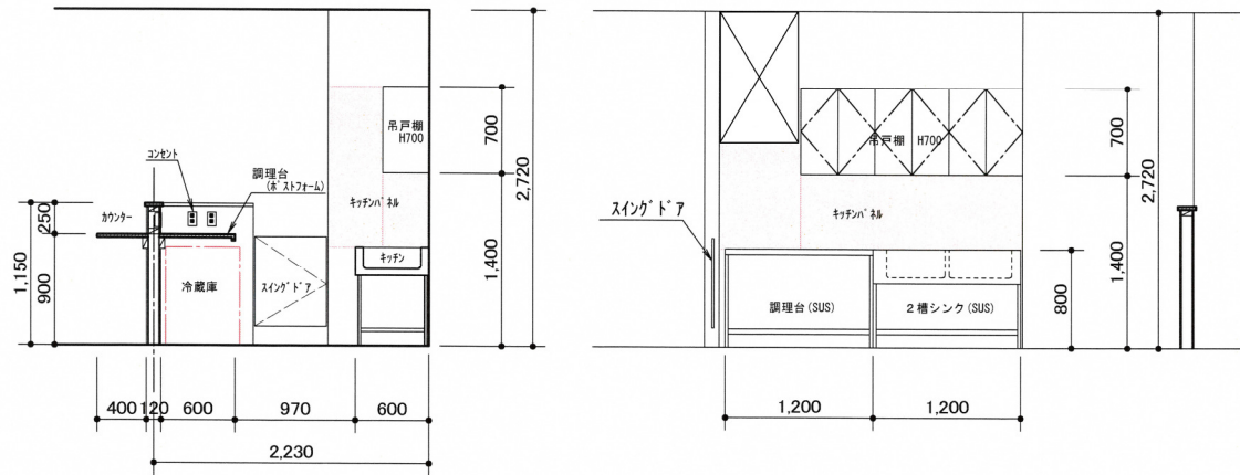
キッチン廻り図面
