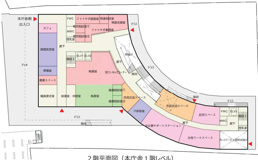
2階平面図 (本庁舎1階レベル)
