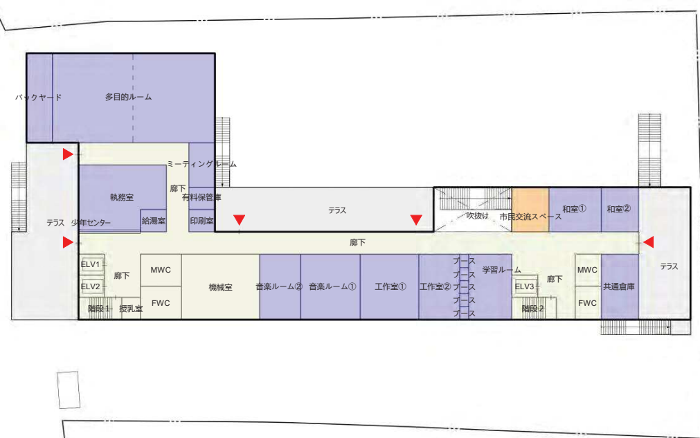
3階平面図 (本庁舎2階レベル)
